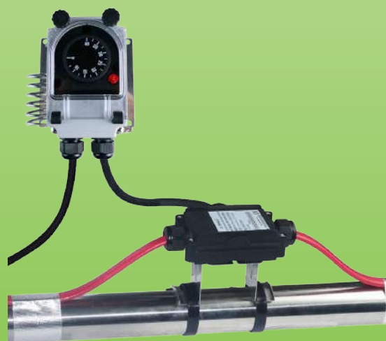
在两根伴热电缆的组装示例，带 Y27 接线盒，用于钢管的防冻保护
