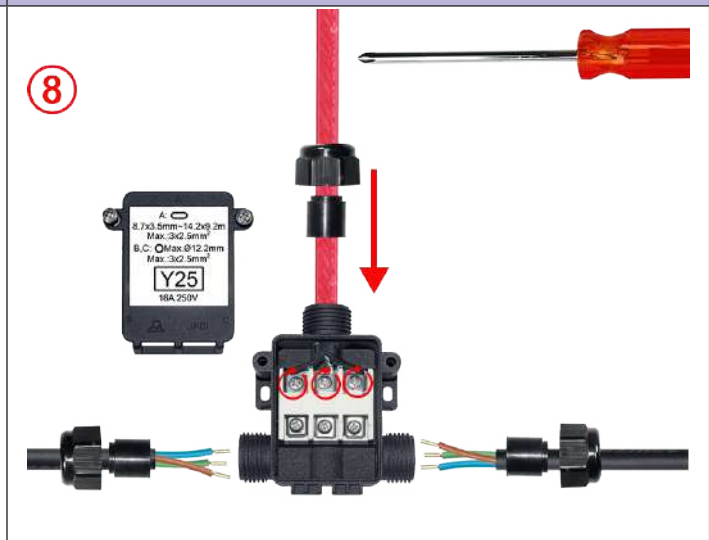
8: 将发热电缆导体的剥皮部分插入到端子，并用螺丝刀拧紧。建议的拧紧力为 1.2Nm。
