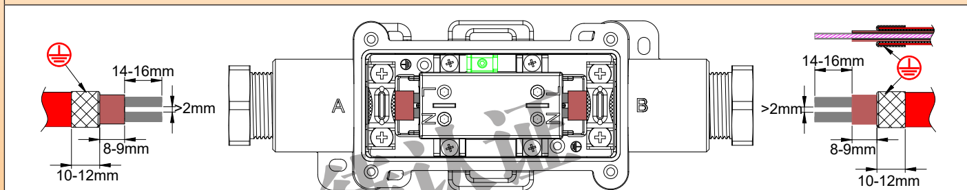
带两根发热电缆的型号
