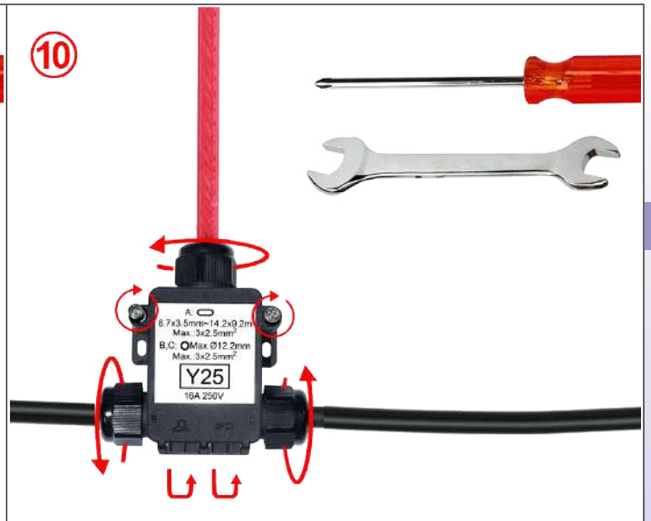
10: 在不转动电缆的情况下，将电缆接头螺母拧入主体，最大的拧紧力度为 3N.m
