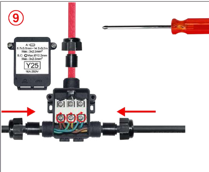
9: 将导体的剥皮部分插入端子并用螺丝刀拧紧。两根导体在各个端子里，在鞍座的每一面上。建议的拧紧力度为 1.2Nm。
